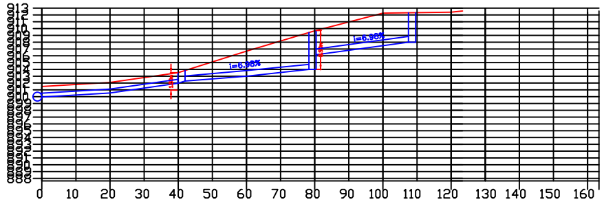
PERFIL LONGITUDINAL ESC: 1:100
