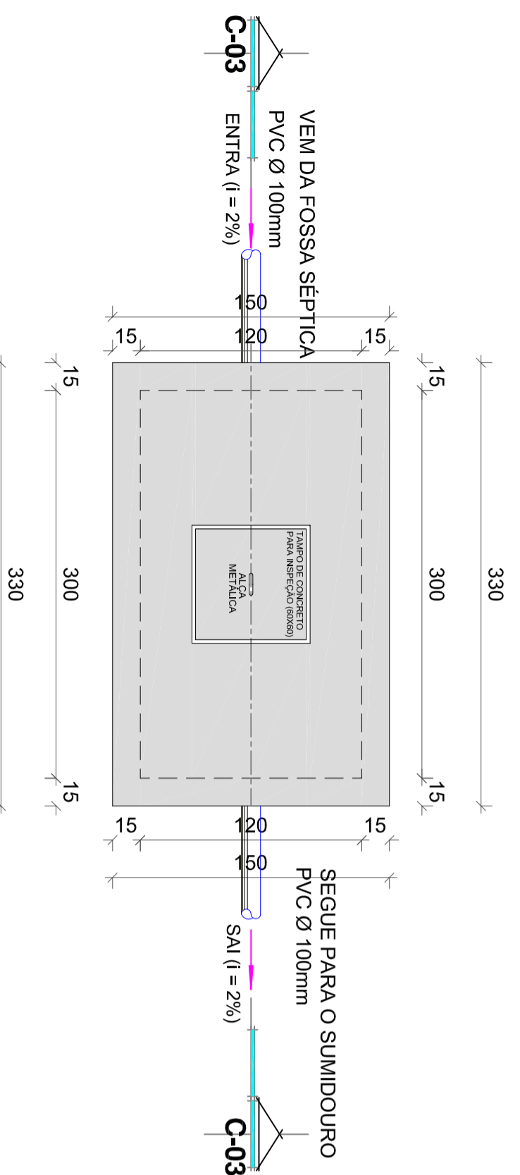
PLANTA BAIXA FILTRO ANAERÓBIO ESCALA 1/20
