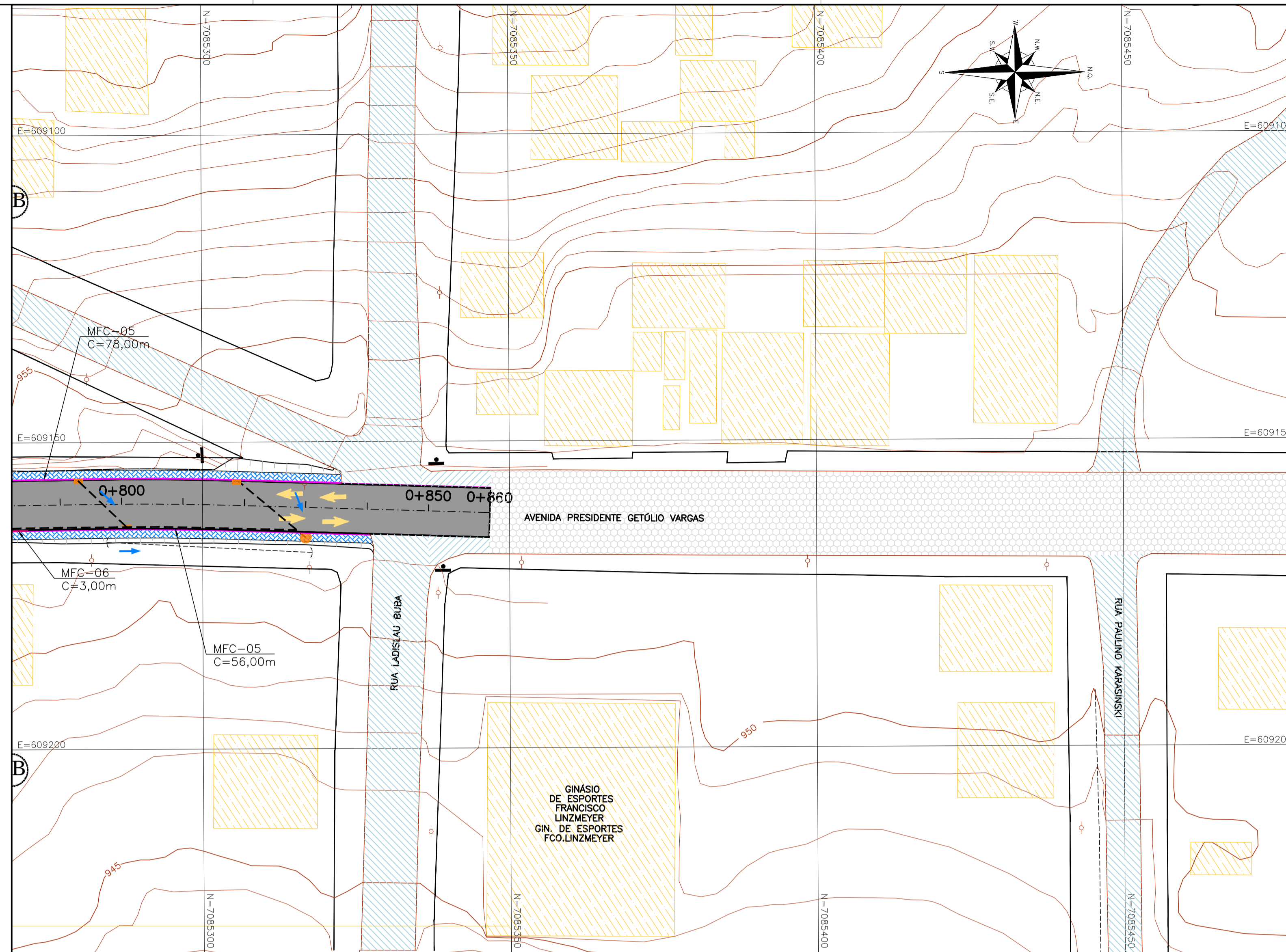
PLANTA DRENAGEM-SUPERFICIAL
